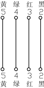
芯线接法(1:1)
